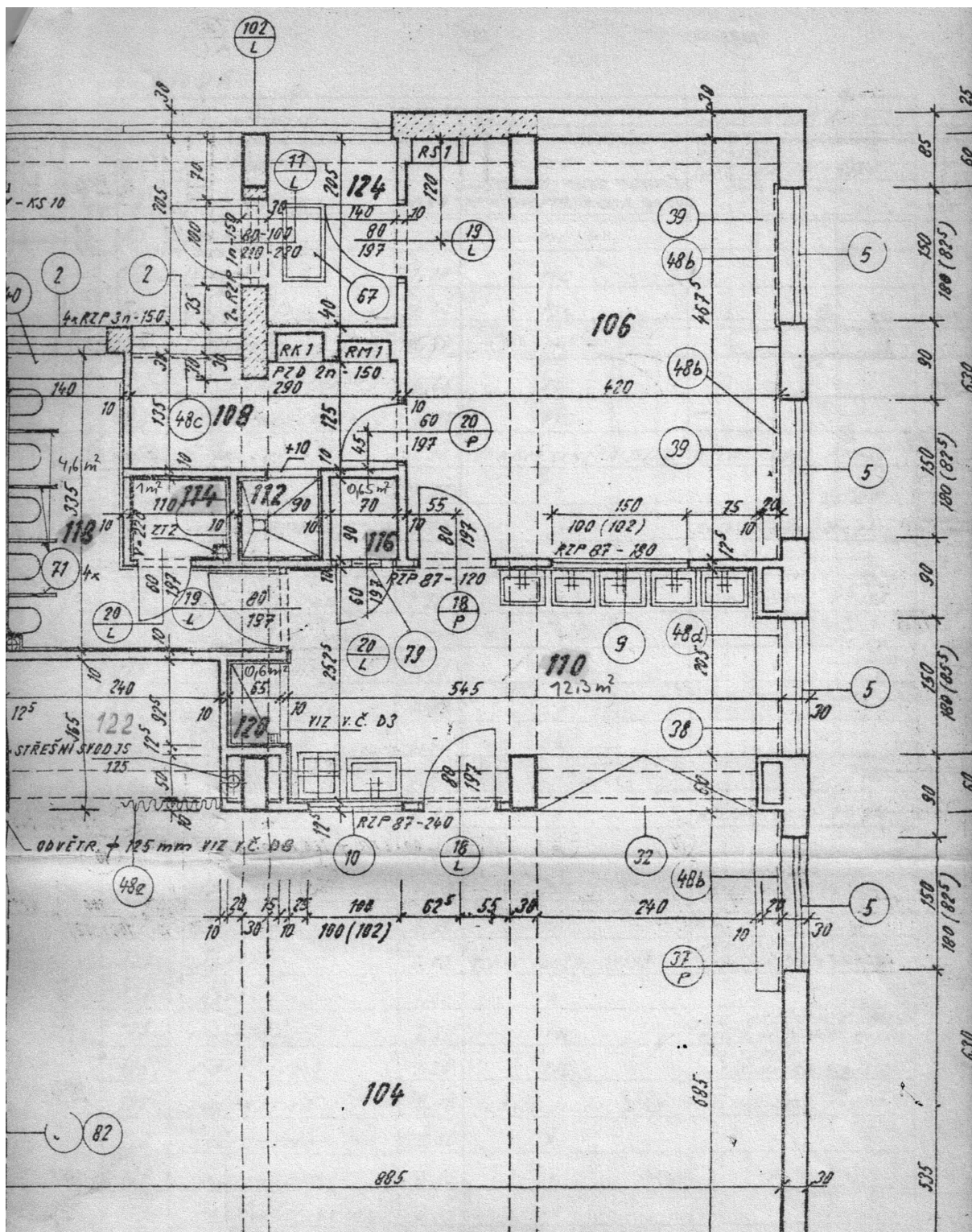
základní schéma soc.zařízení, všechny soc zařízení jsou s podobnou dispozicí
