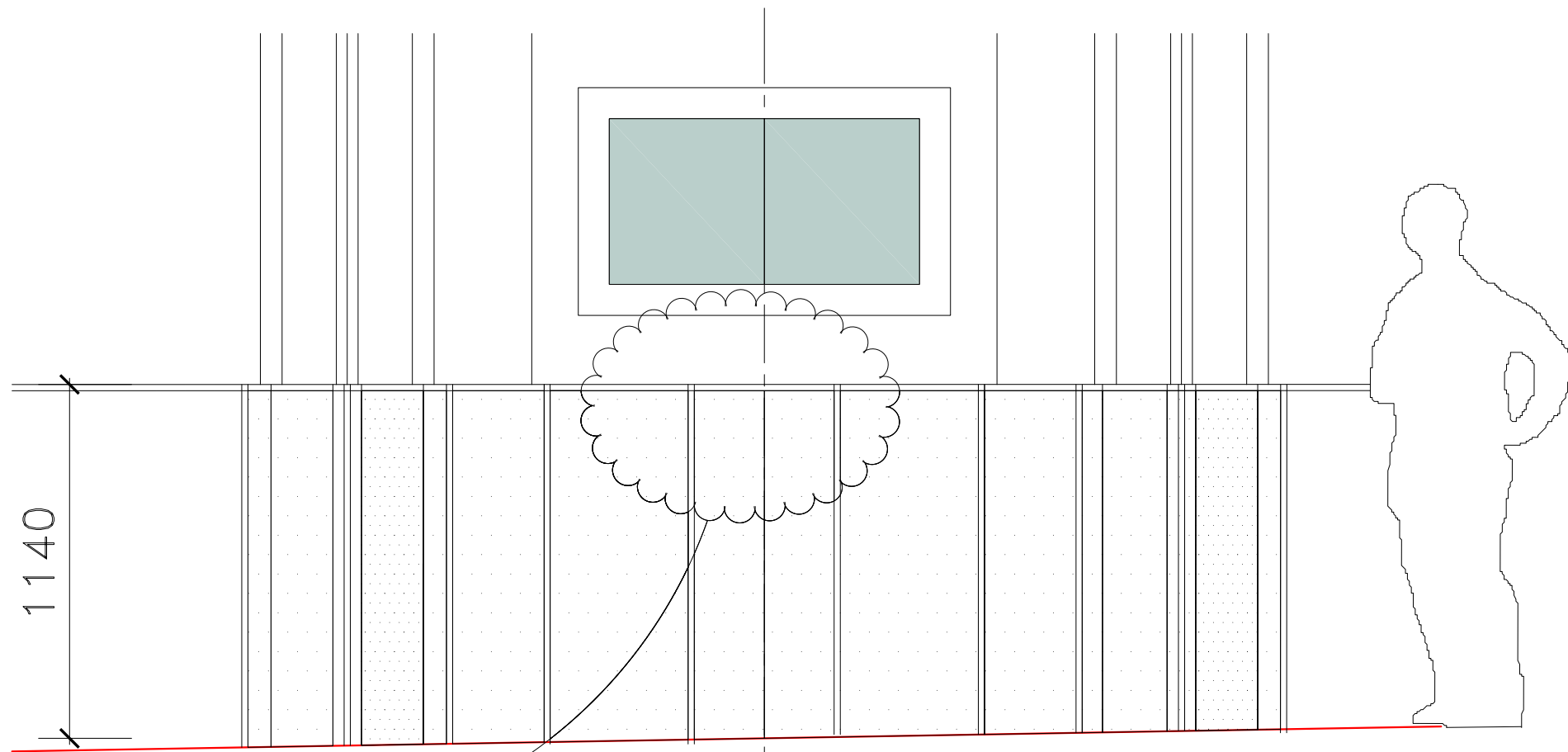
VIZ DETAIL 1:5
